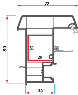
AMS 8006 Hareketli Orta Kayıt Profili Movable Mullion Profile
