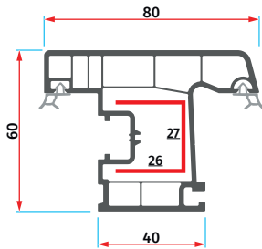
AMS 6031 Dışa Açılır Pencere Kanat Profili Transom Window Sash Profile
