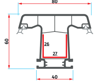
AMS 6019 3 Odacık Orta Kayıt Profili Economic Mullion Profile
