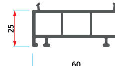
AMS 6032 60'lik Kasa Yükseltme 60 Frame Lift
