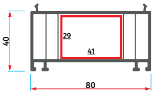
AMS 8013 80'lik Kasa Yükseltme 80 Frame Lift
