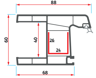
AMS 6034 40'lık U Kasa Profili 40'lık U Frame Profile
