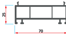
AMS 7024 70'lik Kasa Yükseltme 70 Frame Lift
